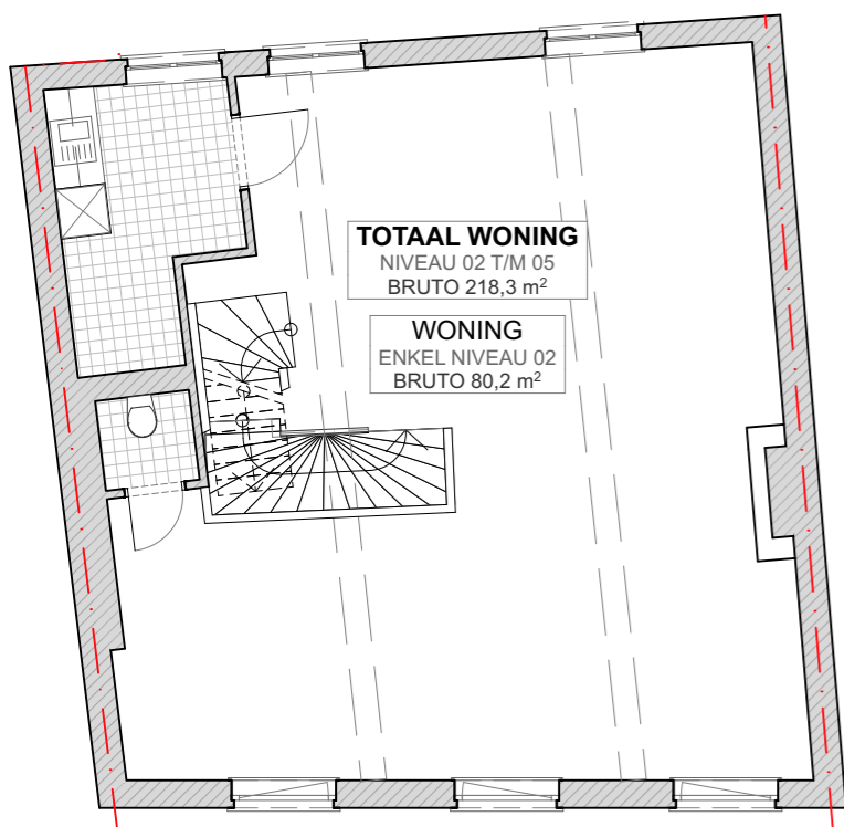
NIVEAU 02 HANDEL + WONING 1:100
