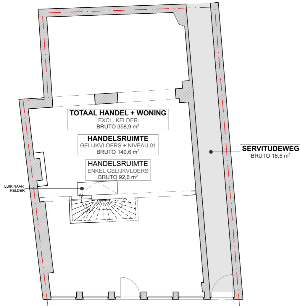
GELIJKVLOERS HANDEL + WONING 1:100
