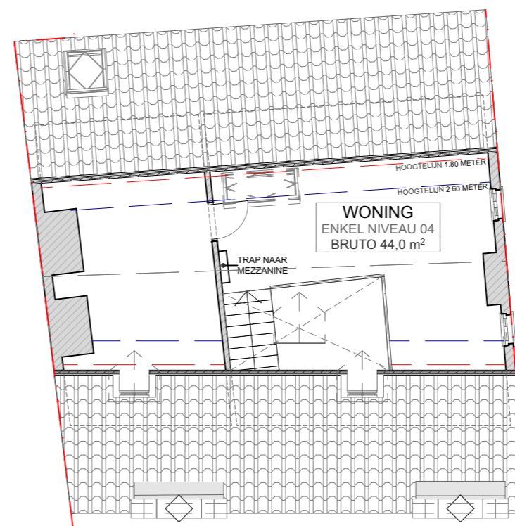
NIVEAU 04 HANDEL + WONING 1:100
