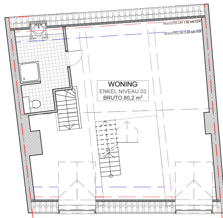
NIVEAU 03 HANDEL + WONING 1:100
