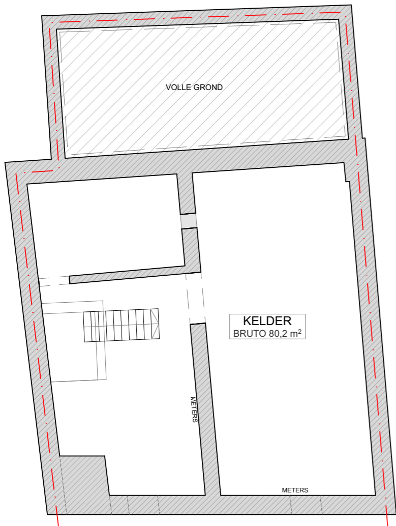
KELDER HANDEL + WONING 1:100
