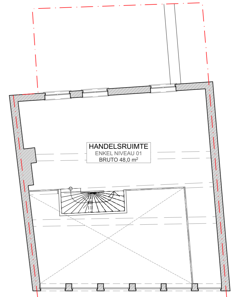
NIVEAU 01 HANDEL + WONING 1:100
