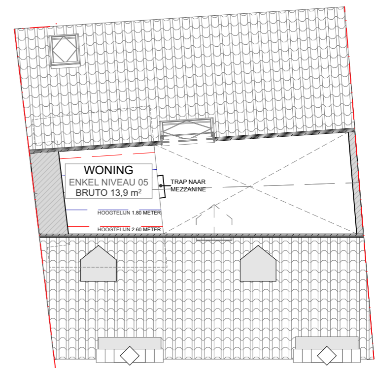
NIVEAU 05 HANDEL + WONING 1:100
